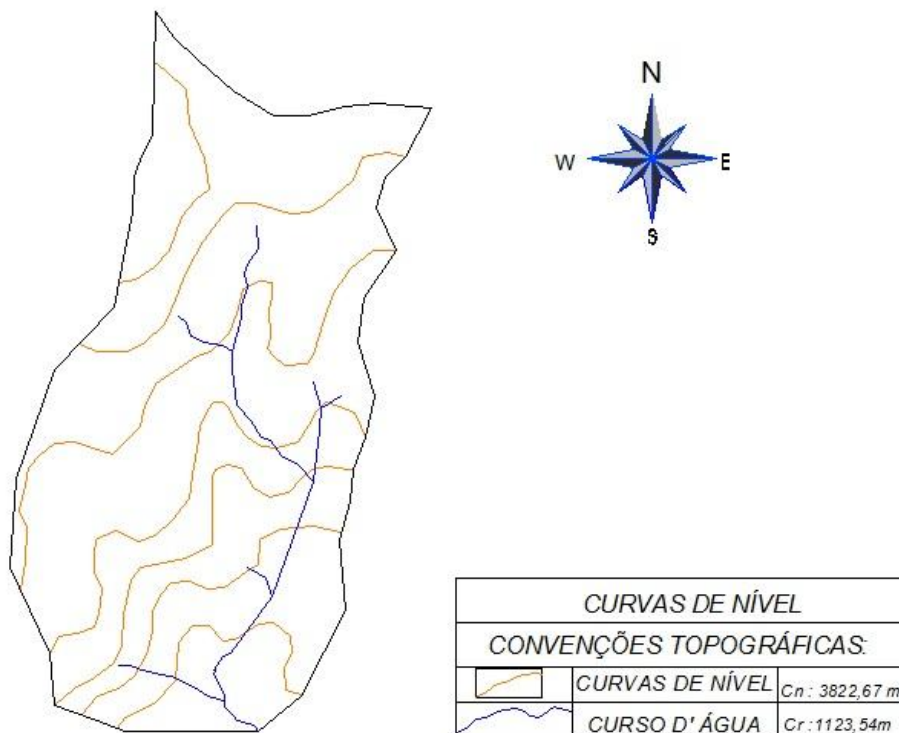
Figura 4 – Curvas de Nível da microbacia do Córrego Barão de Ibitinga
