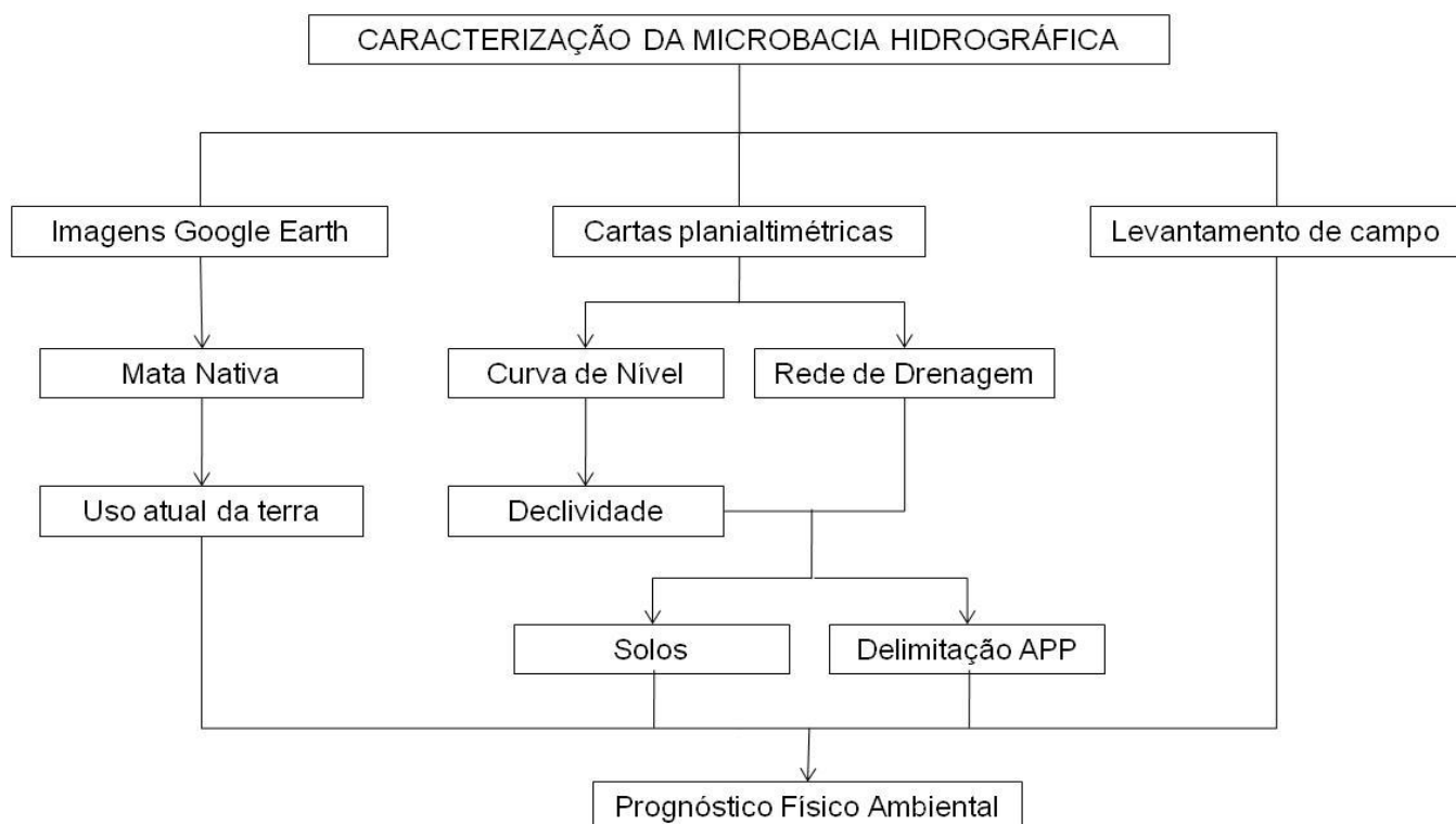
Figura 3 - Roteiro das etapas de trabalho executadas para o prognóstico físico-ambiental da microbacia hidrográfica do Córrego Barão de Ibitinga, no Município de Socorro - SP.
