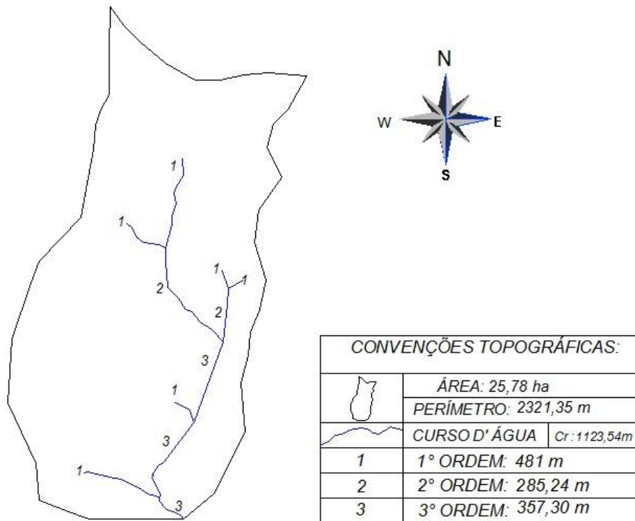
Figura 8 – Ordenamento, Rede de Drenagem e Área da Microbacia Hidrográfica do Córrego Barão de Ibitinga.
