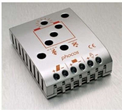
Figura 6.9 – Controlador de carga 12/24 volts 20 amperes
